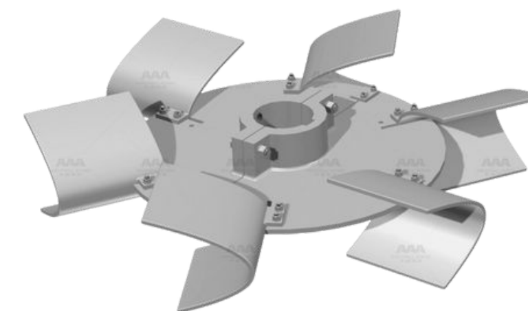
Impellers
